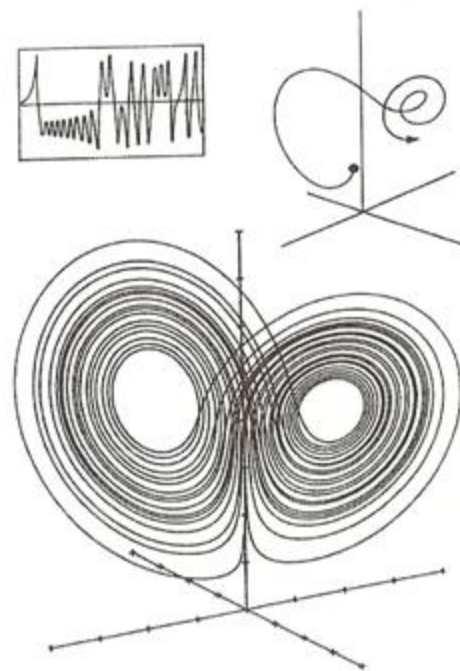
Figura 1 Mariposa de Lorenz
